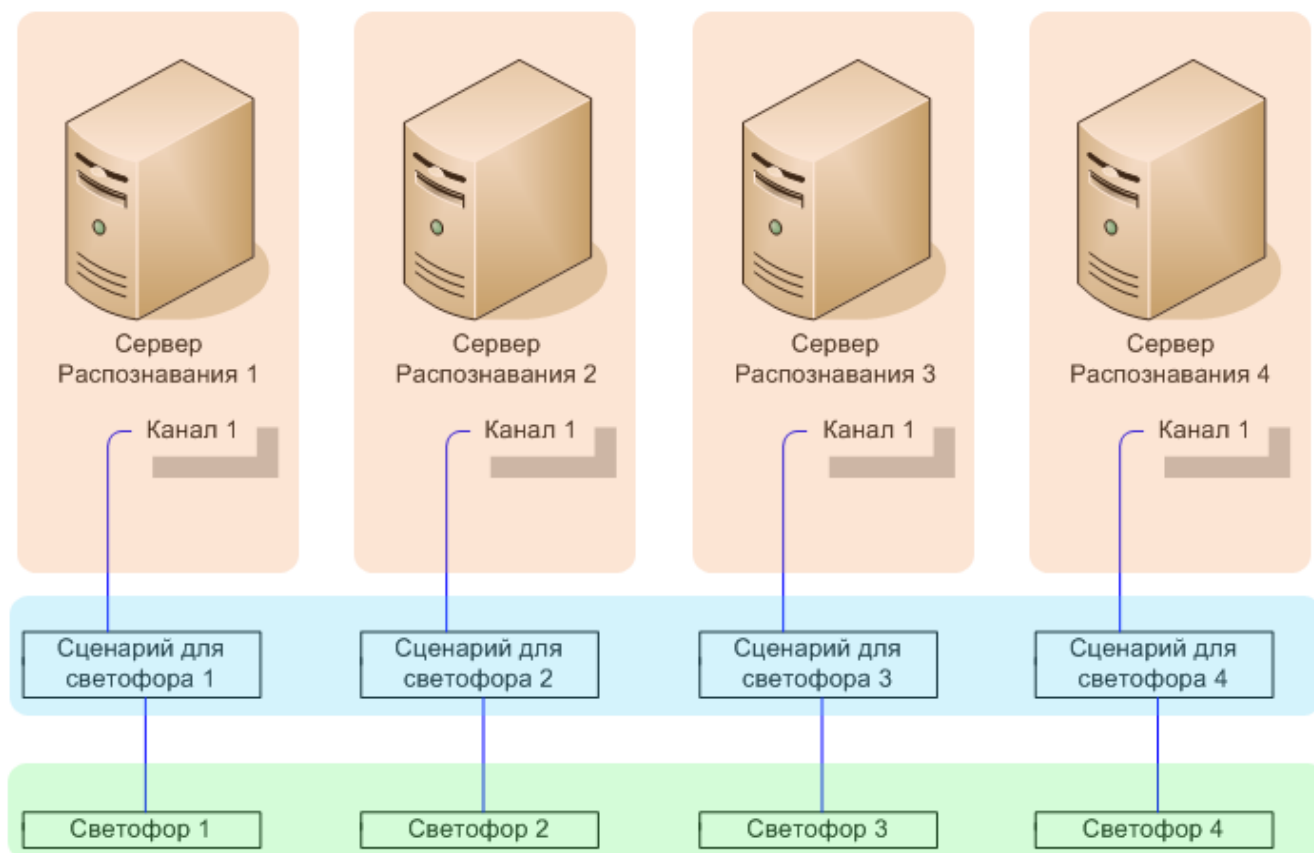
Рис. Схема привязки сценариев обработки к каналам серверов распознавания
