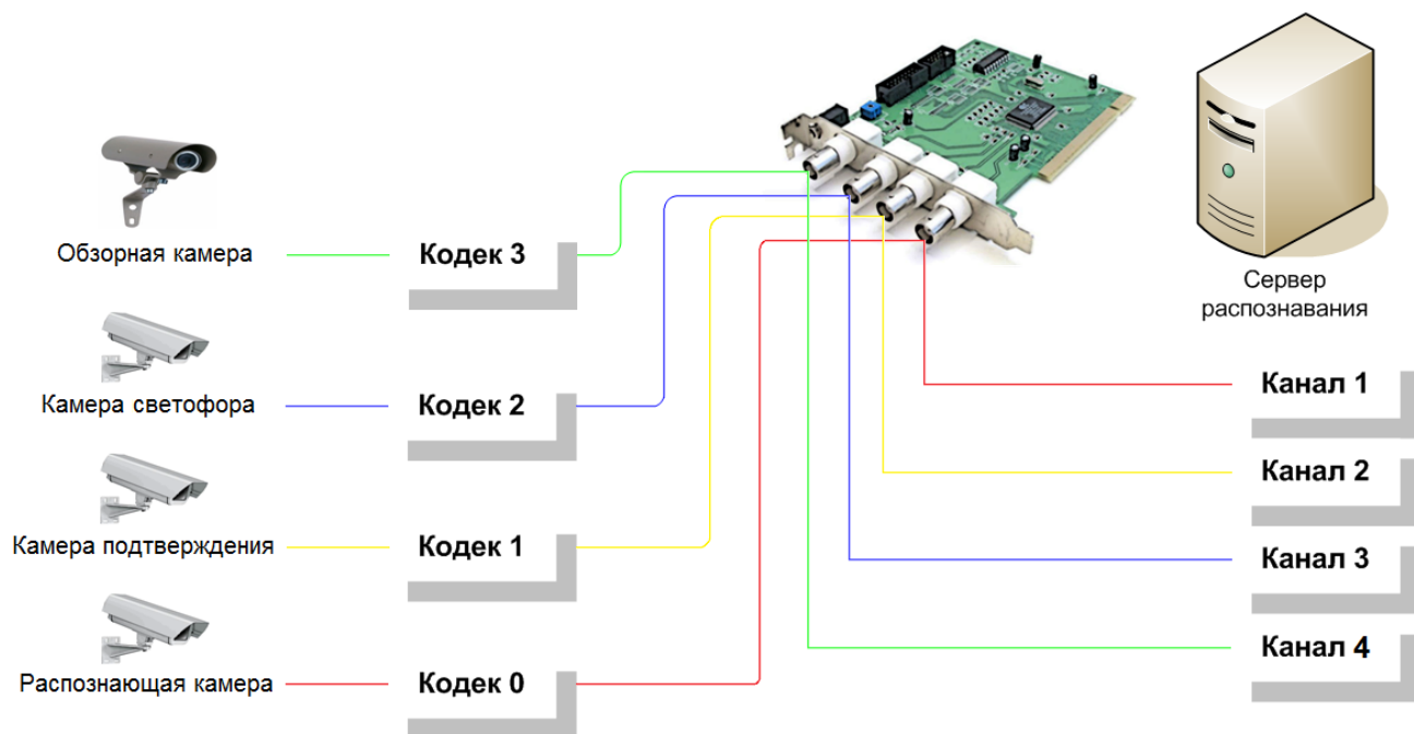
Рис. Схема подключения видеокамер к серверу распознавания
