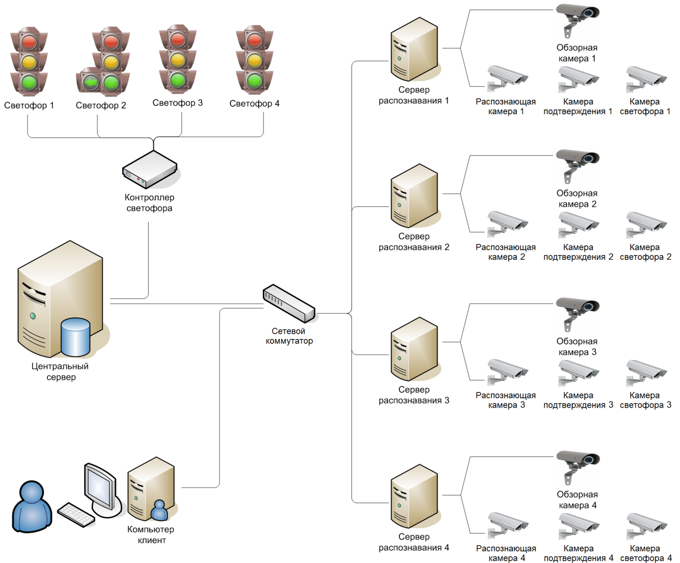
Рис. Общая схема компонентов АПК «АвтоУраган» в конфигурации для перекрестка
